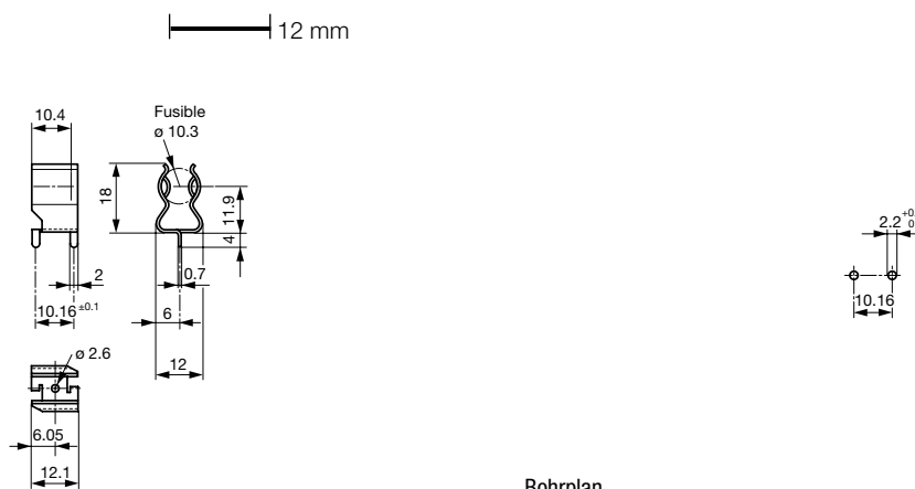
Bohrplan
